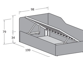
Disegno in versione SX \ Drawing in LH version Sfoderabile \ Removable cover
