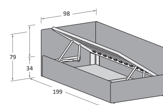
Disegno in versione SX \ Drawing in LH version Sfoderabile \ Removable cover
