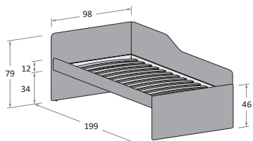
Disegno in versione SX \ Drawing in LH version Sfoderabile \ Removable cover
