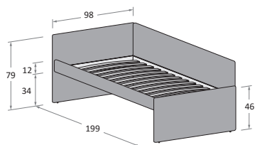
Disegno in versione SX \ Drawing in LH version Sfoderabile \ Removable cover
